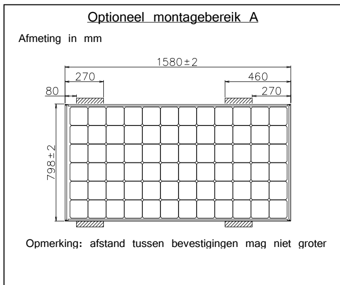
Figuur 1-2: Optioneel montagebereik A
