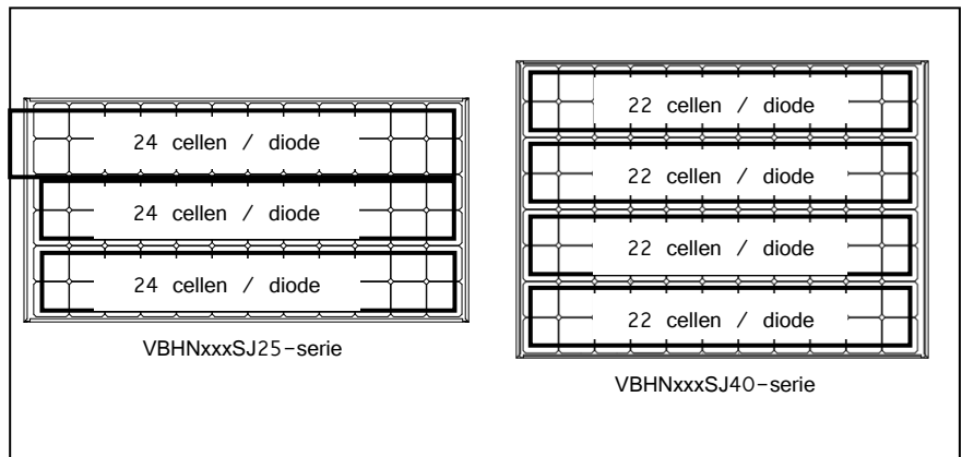
Figuur 4: aantal cellen in serie per omlooptiode
