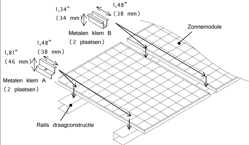
Figuur 6-1 Installatie A
