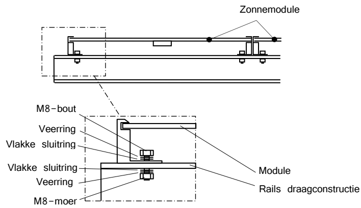
Figuur 6-2 Installatie B
