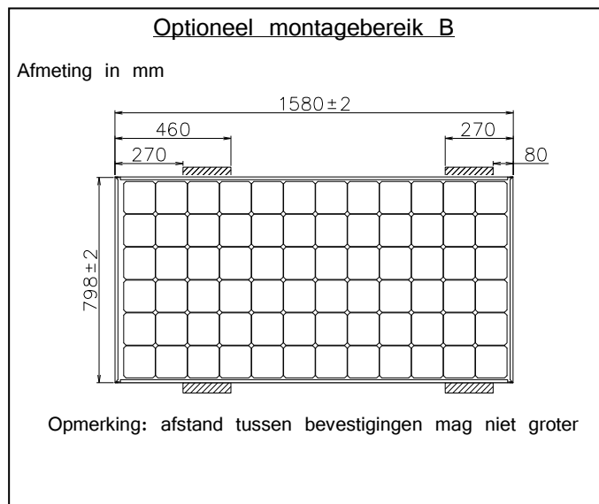
Figuur 1-3: Optioneel montagebereik B
